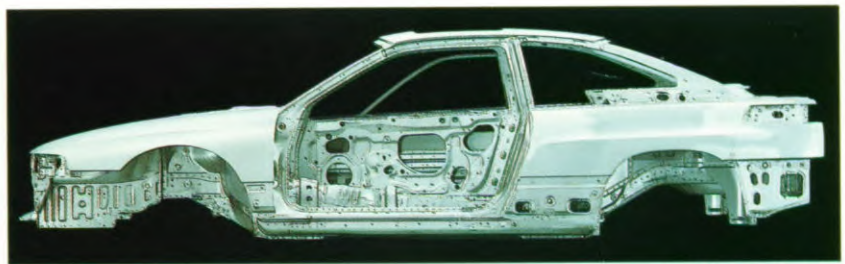
Solide constructie
