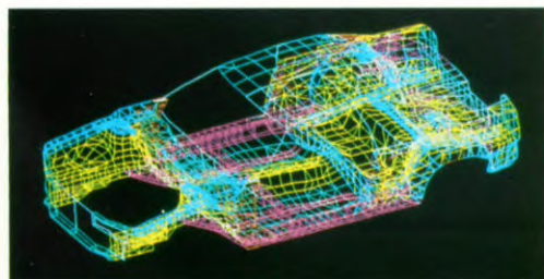
Computeranalyse van de carrosseriestijfheid
