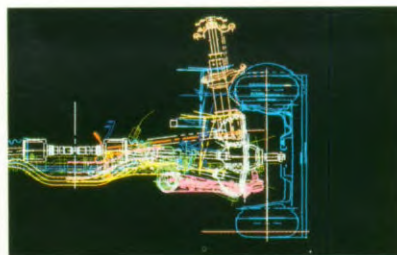
Voorwielophanging
