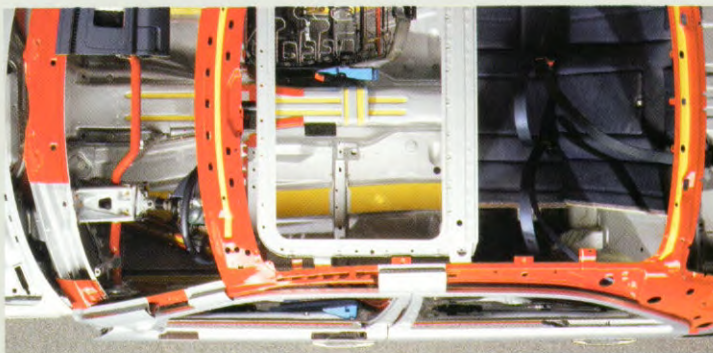
De basis voor de veiligheid in de E-klasse: de zeer stabiele veiligheidskooi.
