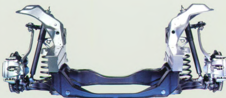
De vooras met dubbele wieldraagarmen verbetert niet alleen de veiligheid en het rijkomfort, maar ook het rijgedrag.
