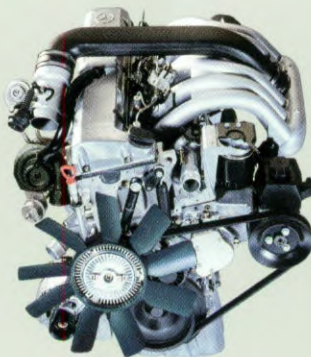
De zuinige vijfcilinder motor met directe inspuiting van de E 290 TURBODIESEL.
