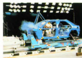
Deceleratie botsingsimulator
