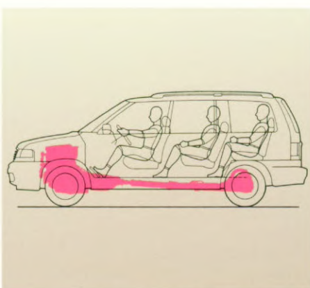
De motor is voorin, in de lengte-as van de auto geplaatst maar de aandrijving geschiedt op de achterwielen voor optimale prestaties en een altijd maximale grip op de weg.
