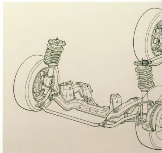
A. Voorwielophanging met MacPherson veerpoten
