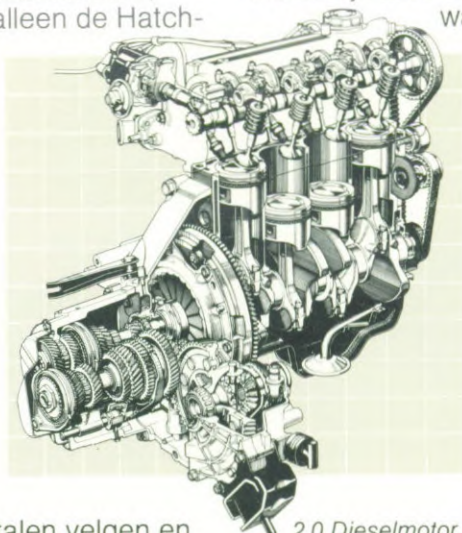
2.0 Dieselmotor.
