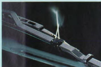
Ruitensproeiers geïntegreerd in de ruitenswiserarmen
