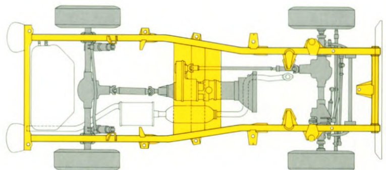
Het stevige chassis van de Jeep Wrangler met z'n rechthoekige balken is beter tegen zware belastingen opgewassen dan traditionele chassis.
