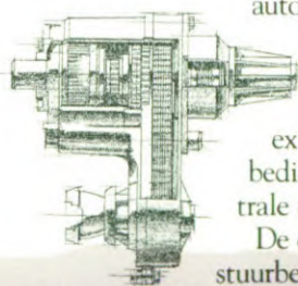
Selec Trac vierwielaandrijving (permanente vierwielaandrijving).
