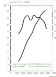
GRAFIEK VAN KOPPEL EN VERMOGEN
