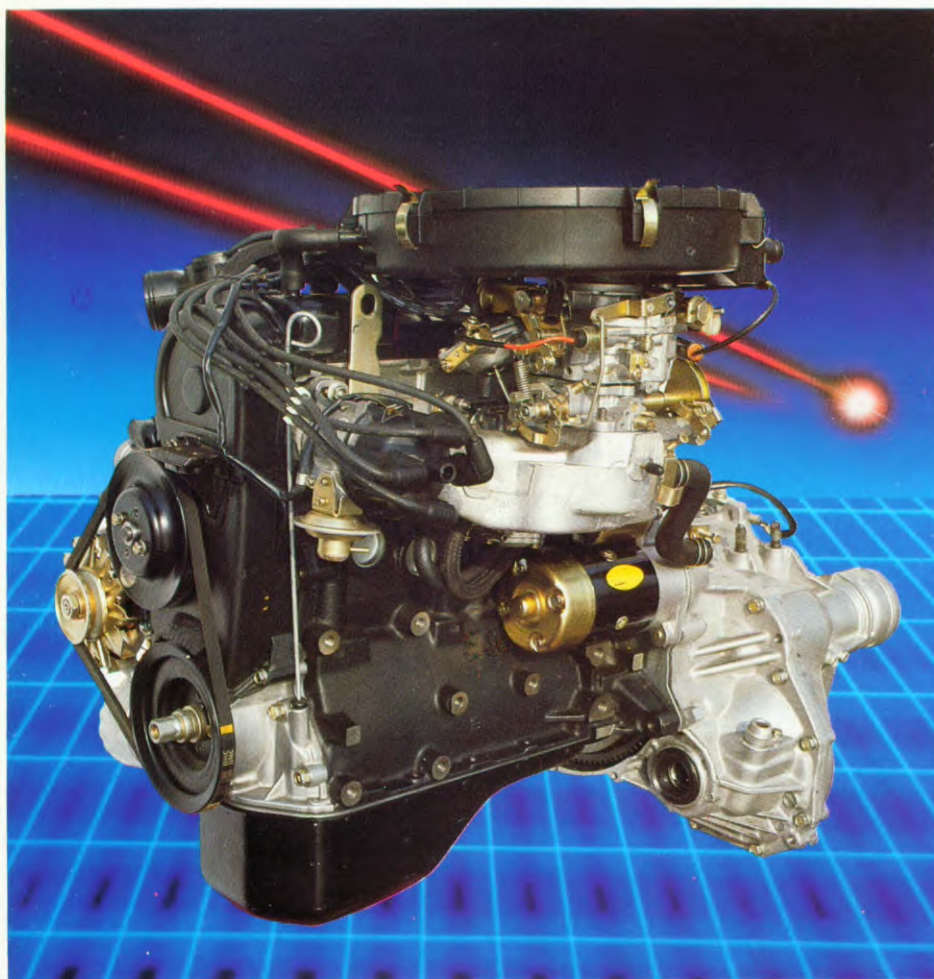
De Pony-motor met bovenliggende nokkenas en elektronische ontsteking. 1500 cm 3 motor van 71 pk bij 5.500 t/min.
