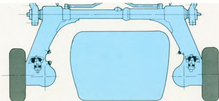
Achterwielophanging met reaktiearmen, schroefveren en stabilisatorstang.
