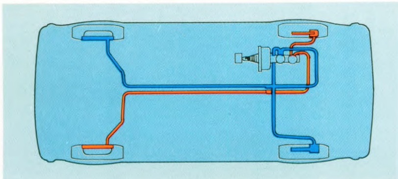
Kruiselings gescheiden remcircuit.
