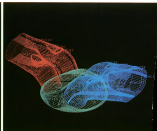
De crossflow opstelling van in- en uitlaatkleppen is in de computer nagebootst en geanalyseerd voor een optimaal motorrendement.
