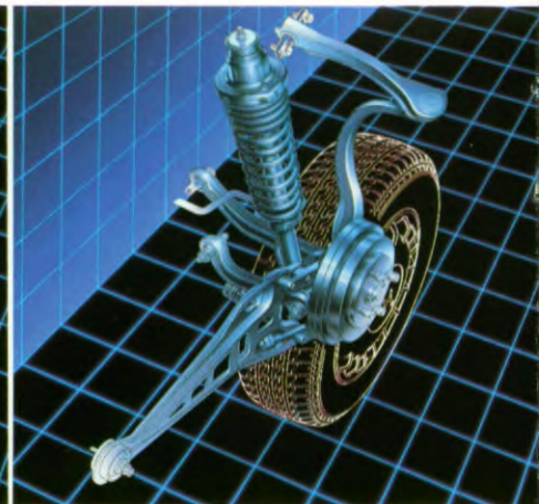
De grotere veerweg van de Double Wishbone achterwielophanging staat garant voor gelijkmatig veercomfort op slechtere wegen, zelfs met volle belading.
