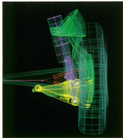
De Double Wishbone voorwielophanging reageert accuraat op alle mogelijke weg- en rij-omstandigheden om een maximale grip van de banden te handhaven.
