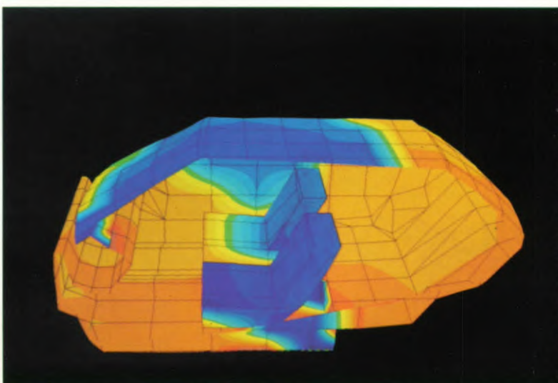
In gedetailleerde ontwerpen van het interieur wijst HANS plekken aan waar isolatie toegevoegd, en geluid van buiten opgevangen kan worden, zodat de inzittenden niet door geluidsoverlast gehinderd worden.
