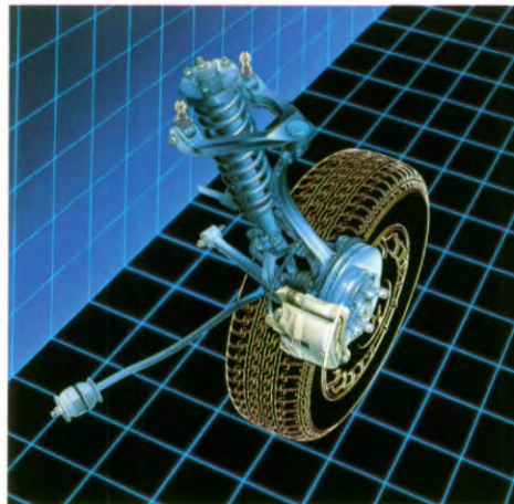
De nieuwe Double Wishbone voorwielophanging neemt alle wielgeleidingskrachten op, zodat de schokdempers een optimaal comfort kunnen waarborgen.
