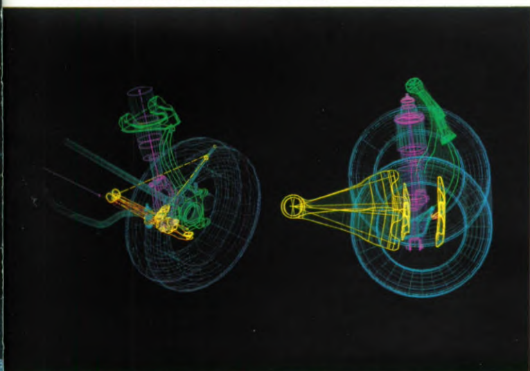
Zowel de voor (links) als achter (rechts) double wishbone wielophanging werden door de computer ontworpen om hun wegrepons nauwkeurig af te stemmen.
