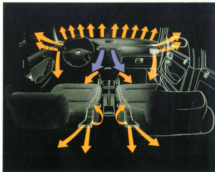
Het krachtige verwarmings- en ventilatiesysteem van de Accord maakt gebruik van een stille twin-blower aanjager (boven) en zorgvuldig gepositioneerde kanalen. Resultaat: een comfortabele luchtcirculatie en optimale luchtverversing.
