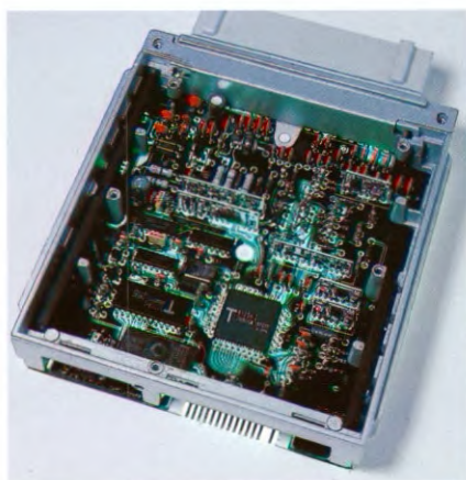
Een blik in het inwendige van de EEC IV elektronische regeleenheid.
