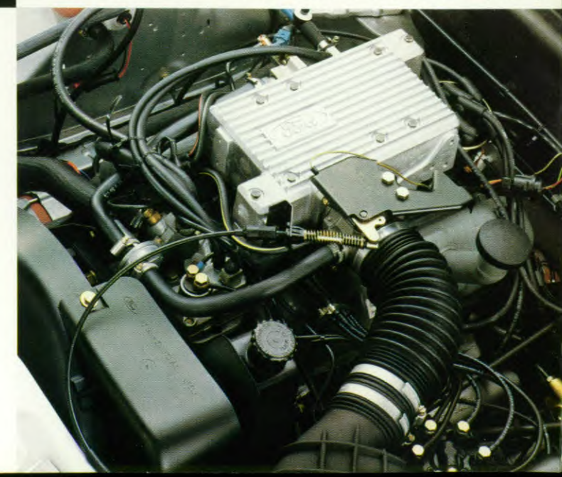
2,8 ltr. V-6 motor met Bosch-K-Jetronic benzine-inspuiting
