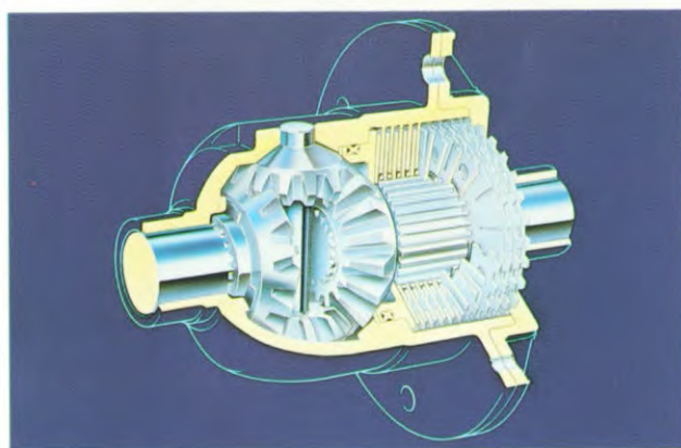
Zelfblokkerend differentieel met viscoskoppeling
