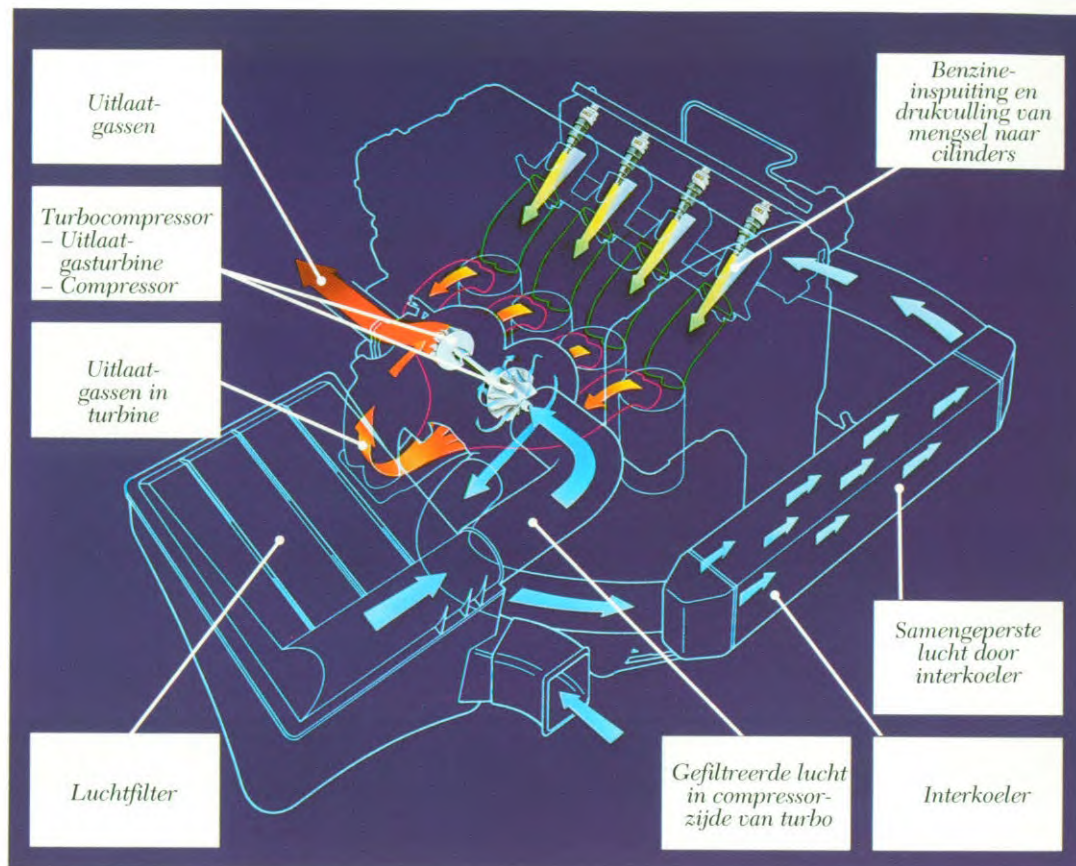
Schema van de drukculling d. m. v. een turbocompressor
