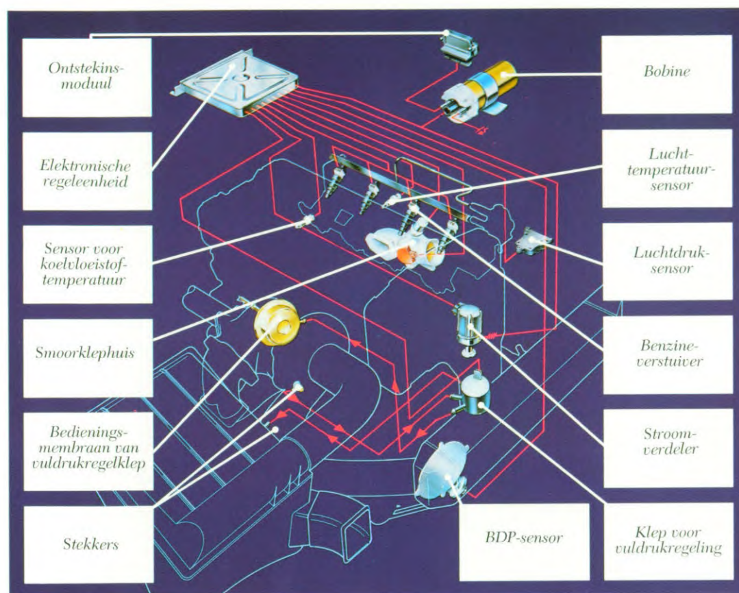
Elektronisch motorregelsysteem
