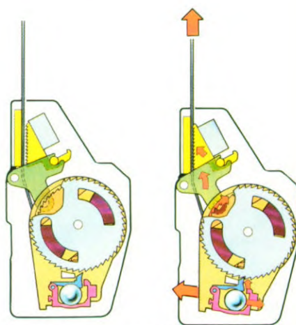
De gordelklampen van de Scorpio.
