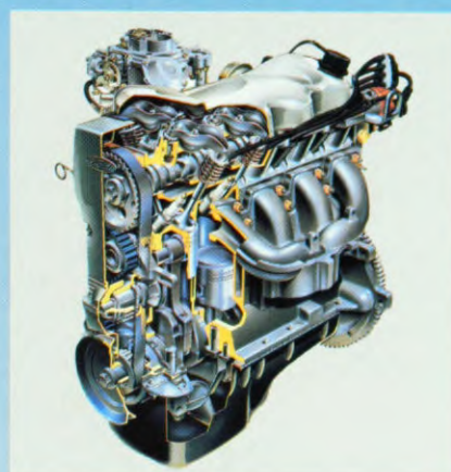
De nieuwe 1.4 CVH motor.
