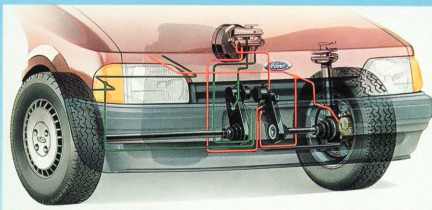
Het nieuwe anti-blokkeer remsysteem heeft een sensor in beide remcircuits van de Orion.
