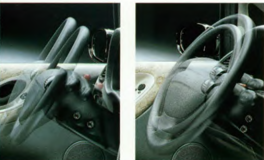
De stuurkolom in de Galaxy is axiaal en verticaal verstelbaar.
