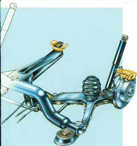
De getrokken geleide-armen van de achterwielophanging zorgen voor een sublieme wegligging.
