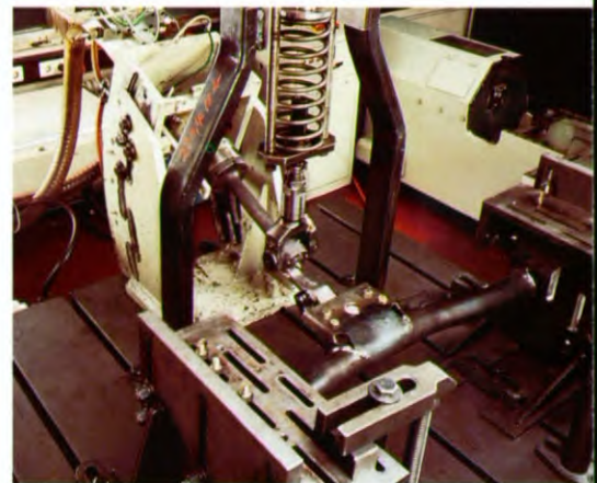
Steekproefsgewijs worden trekhaaken van de productielijn twee miljoen keer onderworpen aan trek- en duwkrachten om ze te testen op zwakke plekken en haarscheurtjes.
