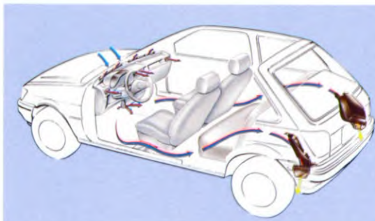
Onbelemmerde toevoer van warme lucht naar de achterpassagiers.
