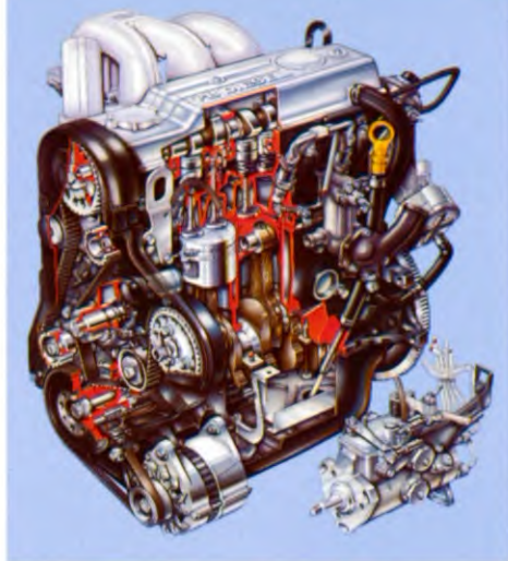
De 1,4 liter CVH-motor met 71 pk/52 kW.
