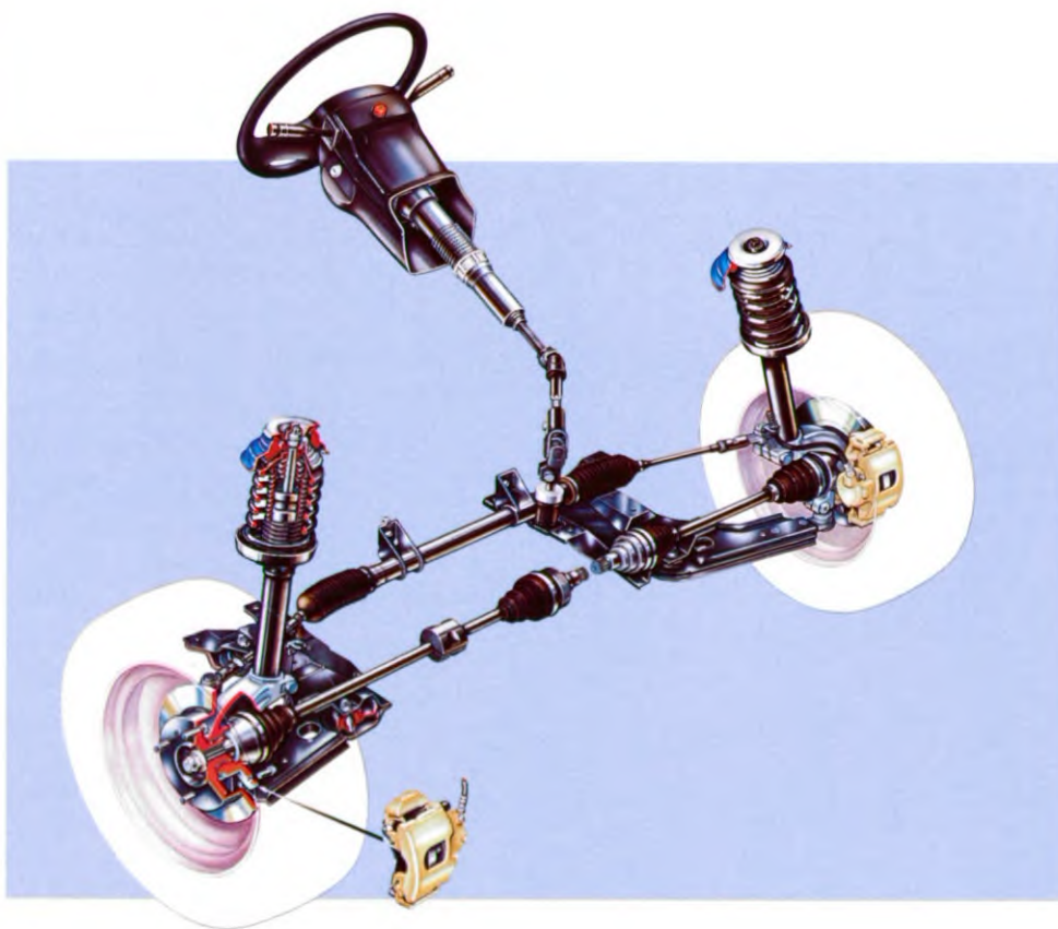
De voorwielophanging en stuurinrichting.
