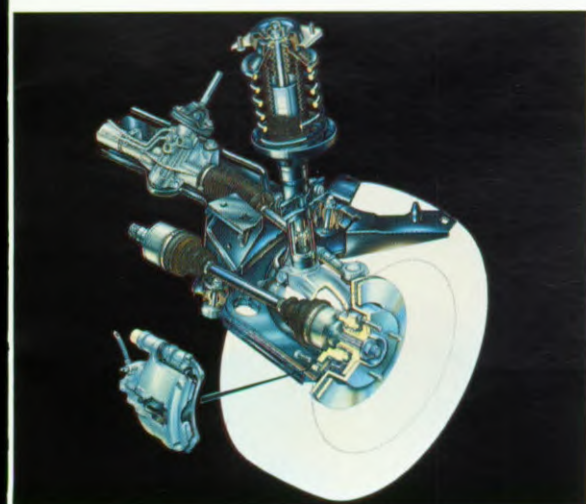
Stuurinrichting met variabele overbrengingsverhouding.
