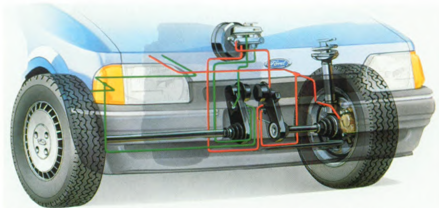
Het nieuwe anti-blokkeer remsysteem heeft een sensor in beide remcircuits van de Escort.
