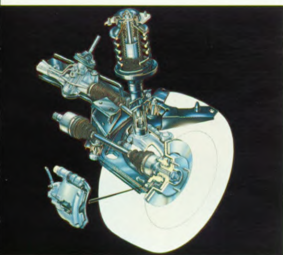
Stuurinrichting met variabele overbrengingsverhouding.
