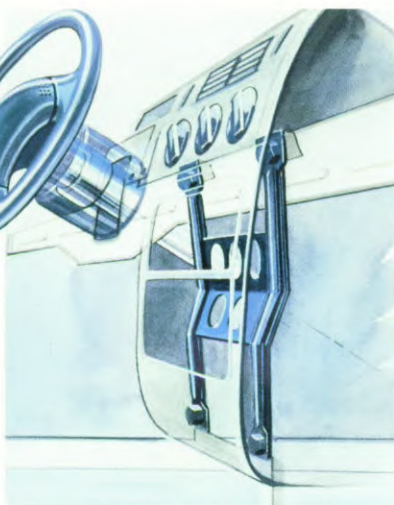
Verticale verankering van de stuurkolom.
