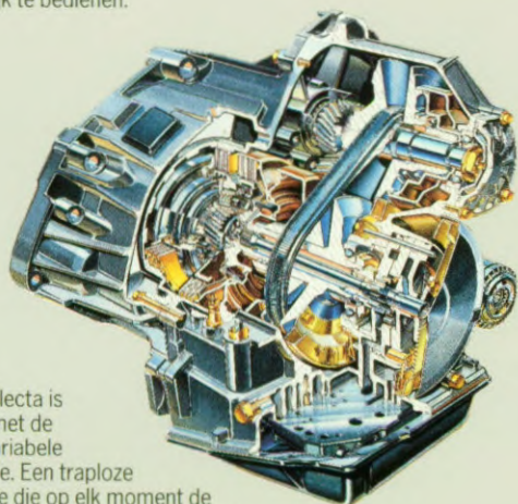
Moderne handgeschakelde transmissie met vijf versnellingen. Soepel en gemakkelijk te bedienen.
