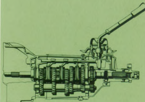
Versnellingsbak
