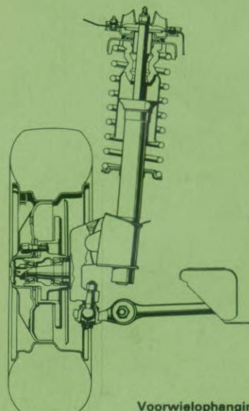
Voorwielophanging
