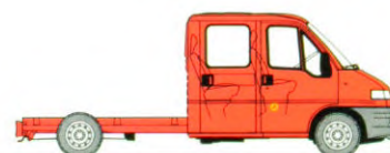
Wielbasis 3,70 m
