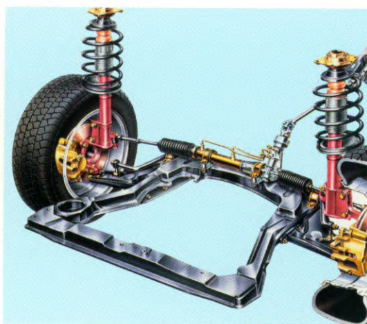
De 'silent blocs' tussen het frame, waarop de achterschokdempers gemonteerd zijn, en het chassis, reduceren trillingen tot een minimum.
