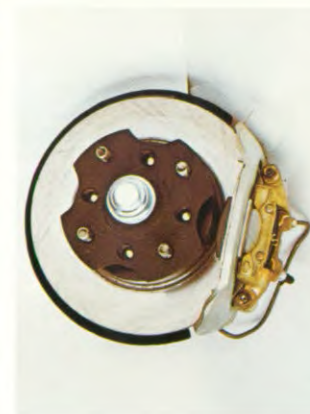
Het remsysteem van de Datsun Sunny Traveller laat zelfs voor de meest verwendende autorijder niets te wensen over. Grote schijfremmen op de voorwielen, rembekrachtiging, gescheiden remsysteem en een remkrachtbegrenzer op de achterwielen, zorgen voor een optimale veiligheid.
