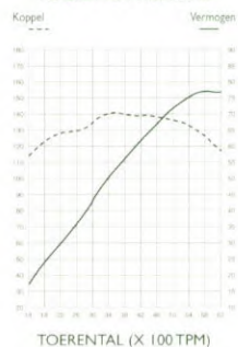
1.6 DOHC PRESTATIE
