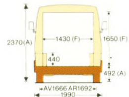
C35 gesloten bestel met normaal dak Lange wielbasis: 4.20 m. Nuttige inhoud: 12,5 m 3 .
