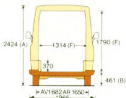
C 25 1300 Gesloten bestel met verhoogd dak Korte wielbasis: 2,923 m. Nuttige inhoud: 7,7 m 3
