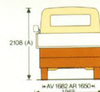
C 25 1300 Pick-up Korte wielbasis: 2,923 m. Enkele cabine
