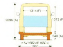
C 25 Combi Korte wielbasis: 2,923 m. Achterbank in normale stand
