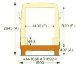
C35 gesloten bestel met verhoogd dak Lange wielbasis: 4.20 m. Nuttige inhoud: 14,3 m 3 .
