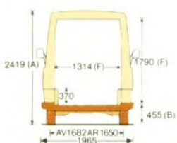
C 25 1300 Gesloten bestel met verhoogd dak Lange wielbasis: 3,653 m. Nuttige inhoud: 10,2 m 3
