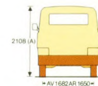
C 25 1300 Chassis Cabine Korte wielbasis: 2,923 m. Enkele cabine
