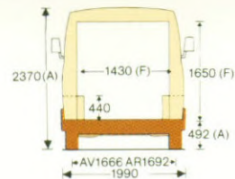
C35 gesloten bestel met normaal dak Korte wielbasis: 3.20 m. Nuttige inhoud: 9,3 m 3 .
