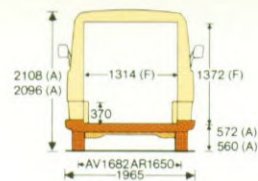
C 25 1000 en 1300 Gesloten bestel met normaal dak Korte wielbasis: 2,923 m. Nuttige inhoud: 6,5 m 3
