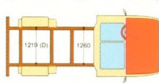
C 25 1300 Chassis Cabine Korte wielbasis: 2,923 m. Enkele cabine
