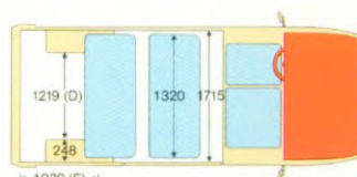
C 25 Combi Korte wielbasis: 2,923 m. Achterbank in normale stand
