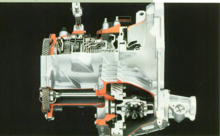
De nieuwe automatische 4-traps transmissie past zich elektronisch optimaal aan de rij-omstandigheden aan.
