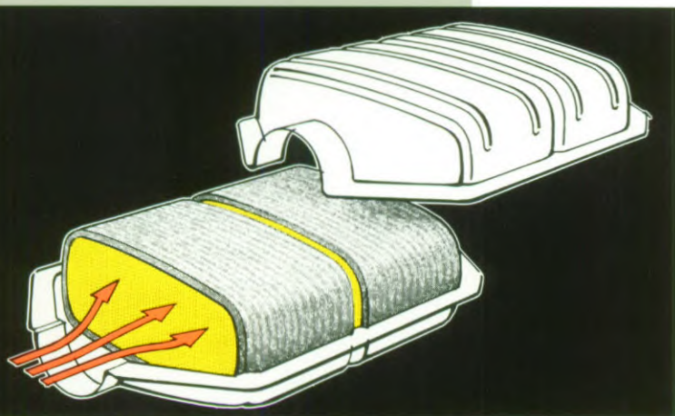
Zoals alle Chrysler-modellen heeft de Voyager standaard een geregelde drieweg-katalysator. Daardoor voldoet hij aan de strenge Amerikaanse milieu-eisen.
