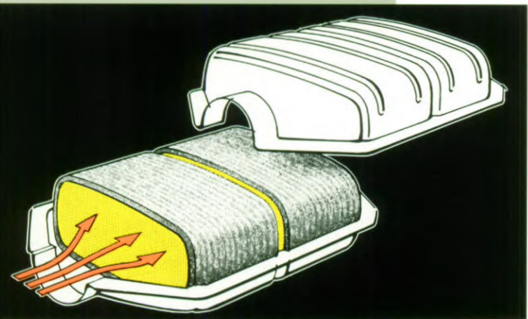
Net als alle andere Chrysler-modellen is ook de Saratoga standaard uitgevoerd met een geregelde drieweg-katalysator.
