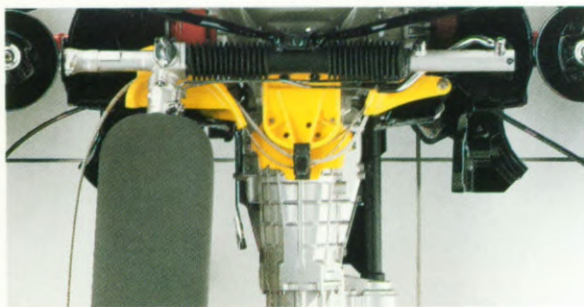
Die Umlenkung für die Stahlseile des procon-ten-Systems.
