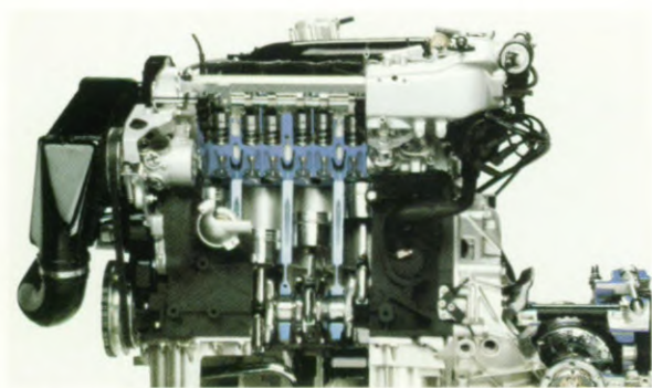
Kraftvolles Durchzugsvermögen durch ein maximales Drehmoment von 309 Nm schon bei 1950/min.
