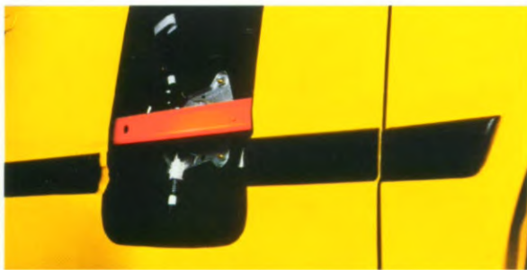
Durch hochfeste Strangpreßprofile in den Türen kann in bestimmten Unfallsituationen die Türverformung erheblich reduziert werden.
