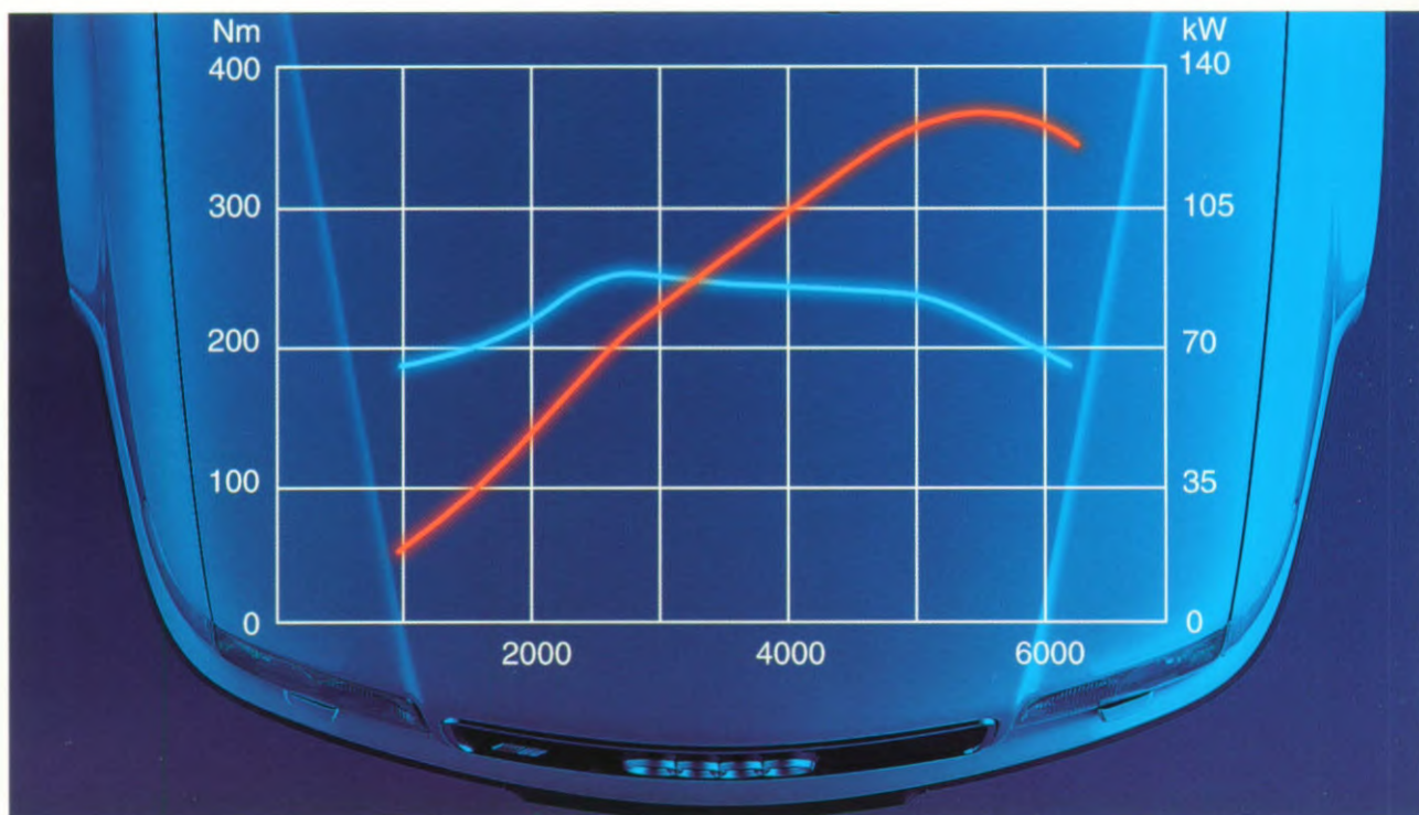
Vermogens- en koppelkrommen van de Audi Cabriolet 2.8E.
