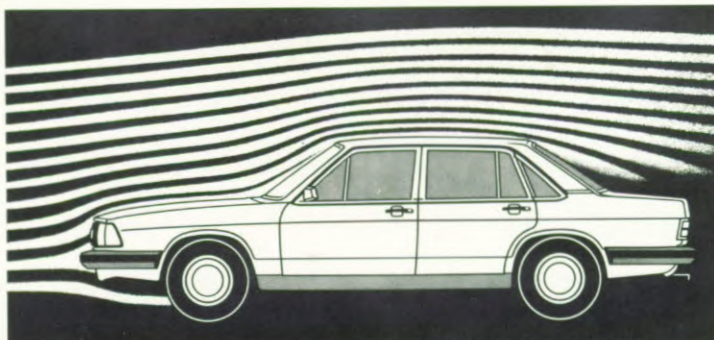
De ideale aerodynamische vorm is het resultaat van langdurige proefnemingen in de windtunnel.
