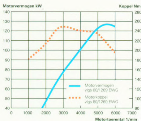
De prestaties van de 128 kW motor.
