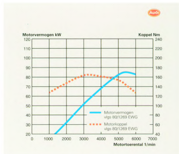
De prestaties van de 85 kW motor.
