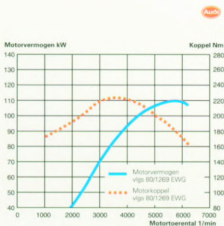
De prestaties van de 110 kW motor.
