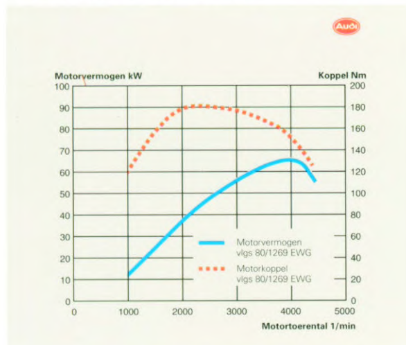
De prestaties van de 66 kW motor.
