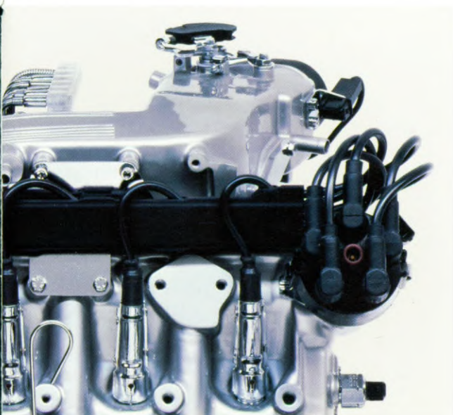
De krachtige 2,3 liter 5-cilinder motor met 98 kW (133 pk).
