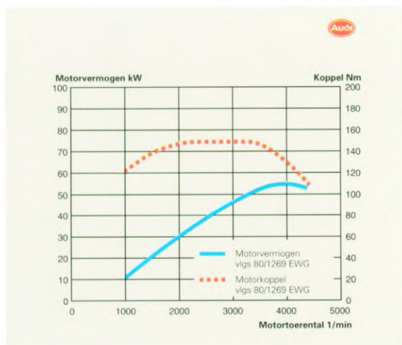
De prestaties van de 55 kW motor.
