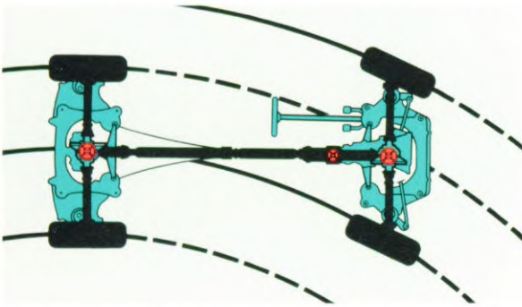
Stabiliteit door het tussendifferentieel, bijvoorbeeld in bochten.
