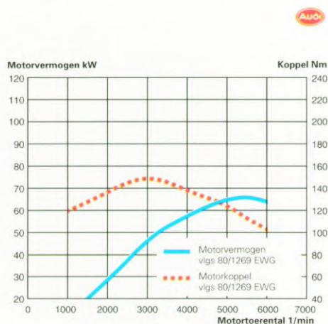
De prestaties van de 66 kW motor.
