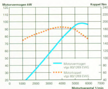
De prestaties van de 98 kW motor.
