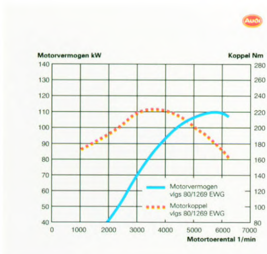
De prestaties van de 110 kW motor.
