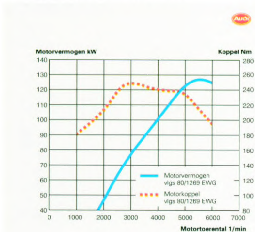
De prestaties van de 128 kW motor.
