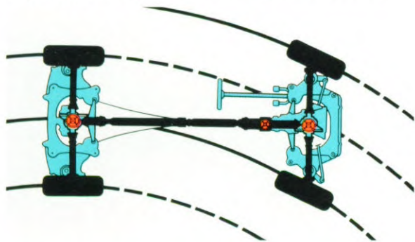
Stabiliteit door het TORSEN-tussendifferentieel, bijvoorbeeld in bochten.
