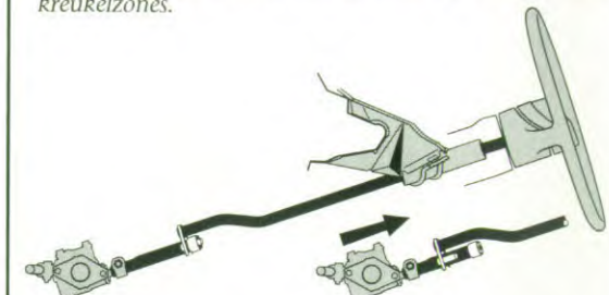
De vervormbare stuurkolom van de Audi 80.
