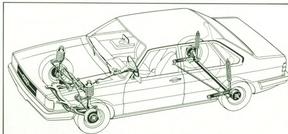
Het geraffineerd geconstrueerde onderstel laat u zelfs de slechtste wegen comfortabel berijden.
