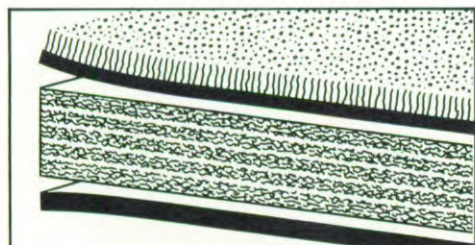
De geluidsisolerende maatregelen in de Audi 80. (Schematisch voorgesteld). Doorsnede van de uit vier lagen bestaande vloerbedekking: (van boven naar onder) 1. tapijt met zwaar-spaat-mat (alleen voorin) 2. vezellaag. 3. bitumen.
