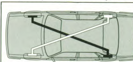
Het diagonaal gescheiden tweekringsremsysteem garandeert een volledig gelijke remkrachtverdeling over voor- en achteras. Ook als er één remcircuit zou uitvallen. Beide assen behouden in dat geval een remkracht van 50%.
