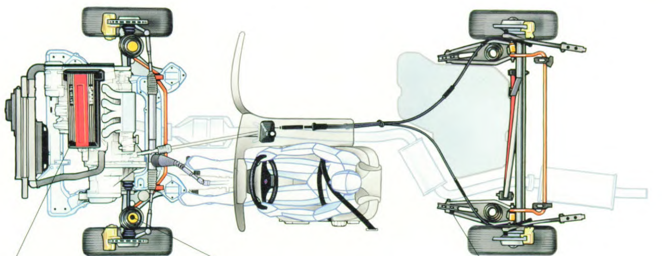
De dwarsgeplaatste motoren de versnellingsbak bevinden zich voor het midden voor de voorwielen.
