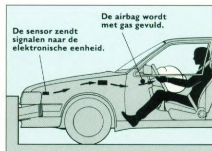
Er zijn 20 milliseconden verstreken sinds het moment van de botsing. De sensoren hebben het systeem geactiveerd en de airbag wordt opgeblazen.
