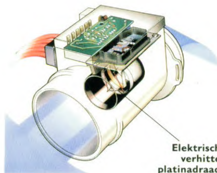
De LH Jetronic luchtstromingsmeter zorgt ervoor dat de motor ongevoelig is voor veranderingen in de omgevingstemperatuur en -druk. De meter heeft geen bewegende delen die aan slijtage onderhevig zijn.
