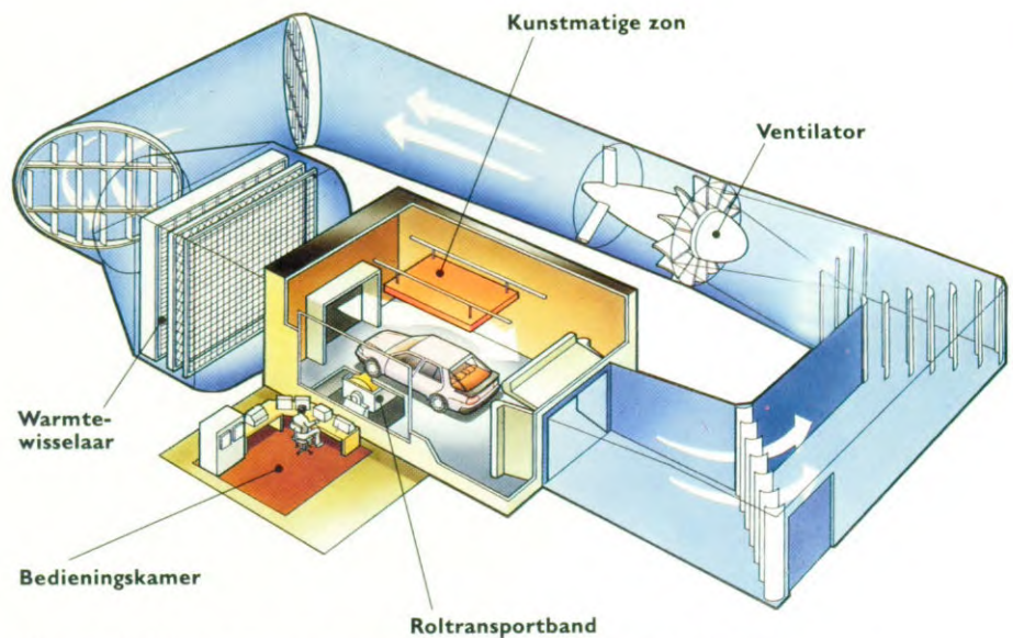
Bijna alle denkbare weersomstandigheden kunnen worden nagebootst in de windtunnel van Saab waarin lichtsnelheden tot 150 km/uur kunnen worden geproduceerd.
