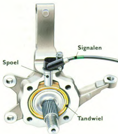
Een ingebouwde vochtbestendige sensor op elk van de wielen registreert de snelheid van elk wiel. De sensor werkt met behulp van inductiestroom – telkens wanneer een van de tanden van een tandwiel de sensor passeert wordt in een spoel elektrische stroom opgewekt.
