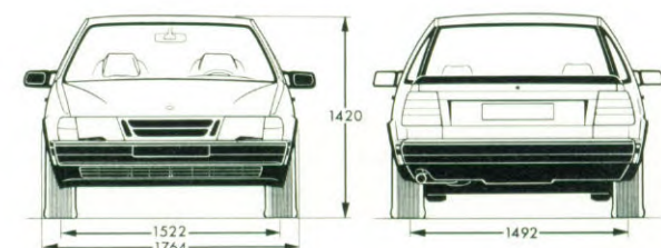
Saab 9000, 5-deursmodellen
