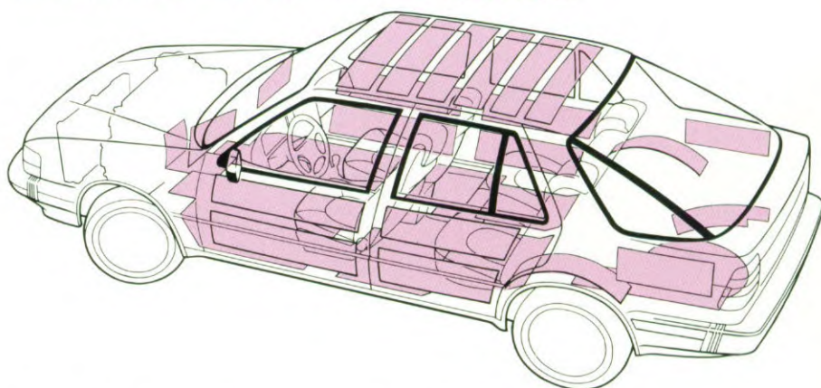
Een dikke laag isolerend materiaal wordt aan het oppervlak van de vloer en de wielkasten gehecht voordat de lak op de carrosserie wordt aangebracht. Op alle plaatstalen oppervlakken, die trillingen zouden kunnen veroorzaken, wordt een geluidsisolerend materiaal aangebracht.
