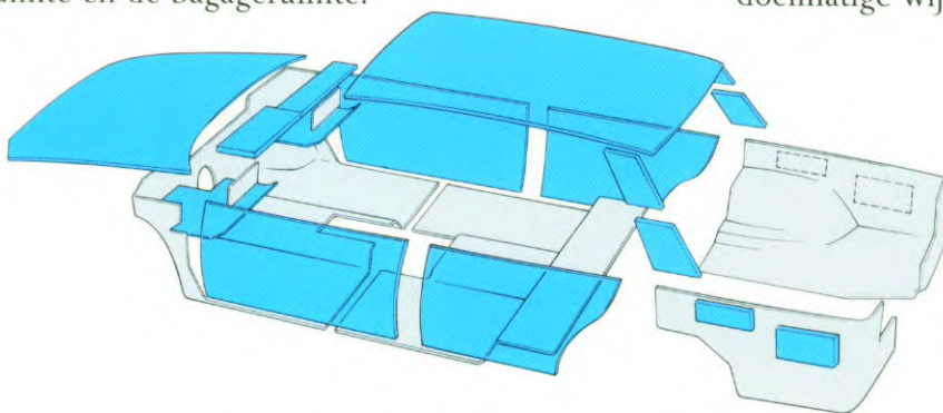
De poreuze, geluidabsorberende materialen die gebruikt worden zijn o.a. schuimplastic en vilt. Deze worden in de motorruimte gebruikt om de geluidsoverdracht van de motor te verminderen en de door de holle ruimten van de carrosserie veroorzaakte resonanties te dempen.
