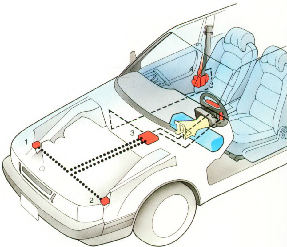
Tenminste één van de twee sensoren (1 en 2) en de veiligheidssensor in de regeleenheid (3) dienen de botsing te registreren alvorens de airbag wordt geactiveerd. Tegelijkertijd spanst de voorspanner (4) de veiligheidsgordel van de passagier naast de bestuurder automatisch aan.
