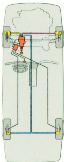
Het Saab ABS+3 systeem heeft drie remcircuits, één voor elk van de beide voorwielen en één voor de achterwielen. Twee geheel onafhankelijke elektronische systemen controleren en vergelijken voortdurend de signalen die zij krijgen.
