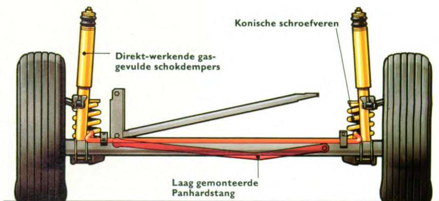
De rechte, starre achteras zorgt ervoor dat zich praktisch geen ongewenste stureffecten voordoen en dat de wegligging fantastisch is. Samen met de vering en de laag gemonteerde Panhardstang wordt tevens voor een hoge mate van comfort gezorgd.
