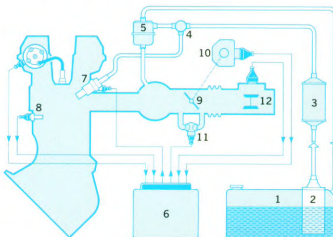
De LH Jetronic luchtstromingsmeter zorgt ervoor dat de motor ongevoelig is voor veranderingen in de omgevingstemperatuur en -druk. De meter heeft geen bewegende delen die aan slijtage onderhevig zijn.
