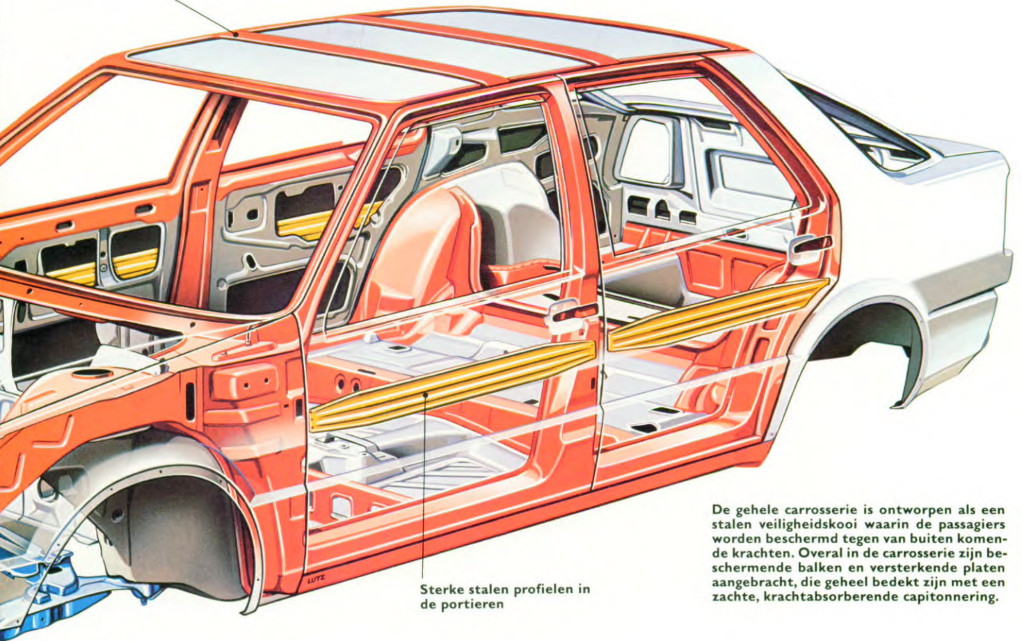
Versterkte dakconstructie
