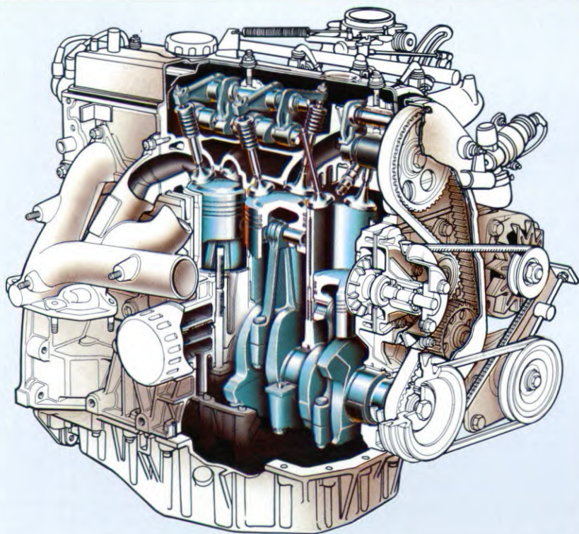
1995 cm³ motor
