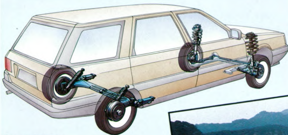
Voor-en achterwielophanging
