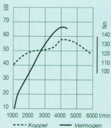
1598 cm 3 motor - 90 pk
