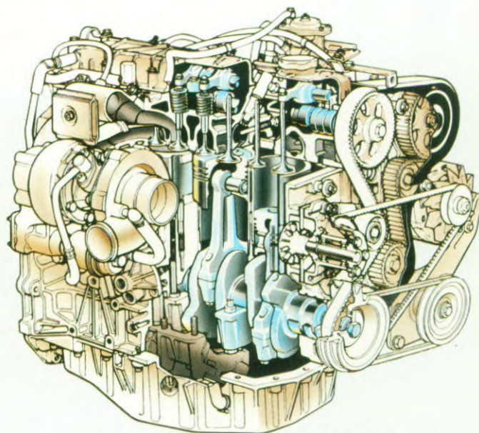
2068 cm 3 Dieselmotor met turbo-compressor
