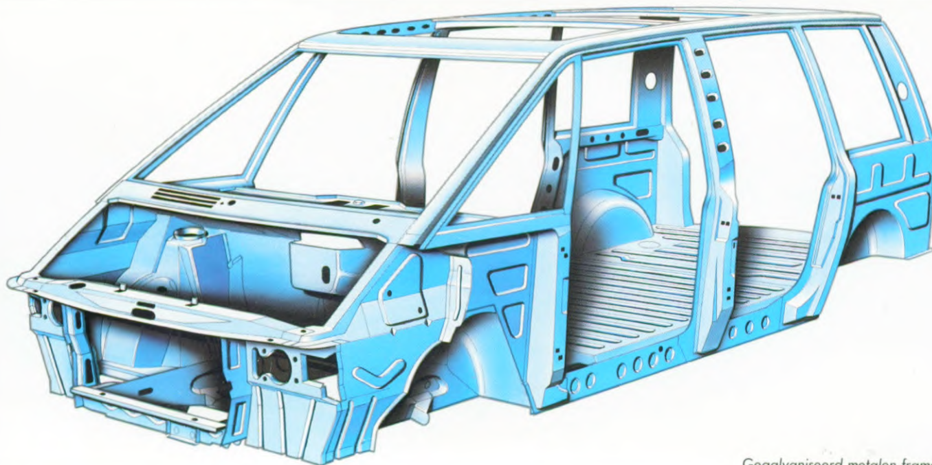
Gegalvaniseerd metalen frame.
