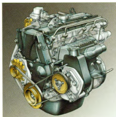
De Sprinter 1,4 liter, 1390 cm 3 , 57,5 kW/80 pk.
