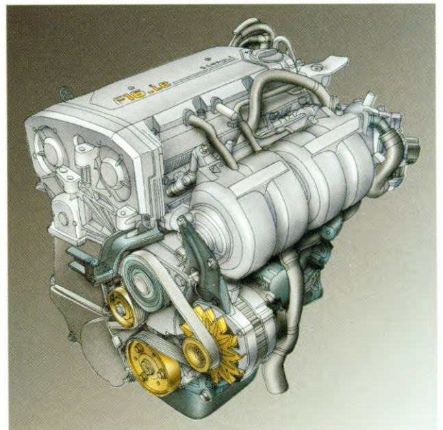
De Super Sportieve 1,8 liter 16V, 1764 cm 3 , 99 kW/137 pk.
