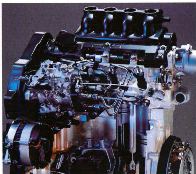
1870 cm 3 dieselmotor.
