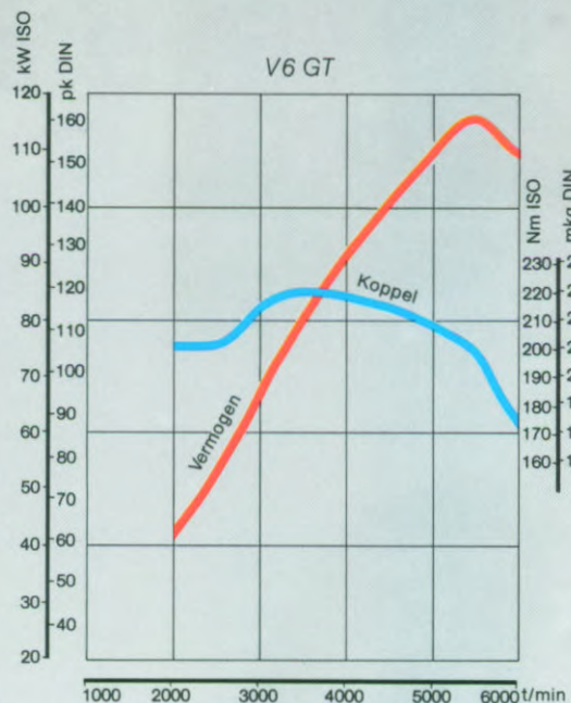
Koppel en vermogenskromme
