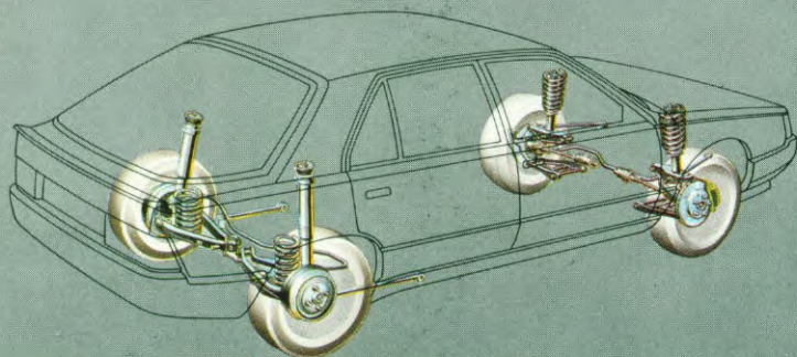
Vering : 4 onafhankelijk geveerde wielen. Voortrein met negatieve stuurstraal en anti-duik geometrie.
