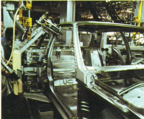
Meting bij assemblage van de portieren door robots
