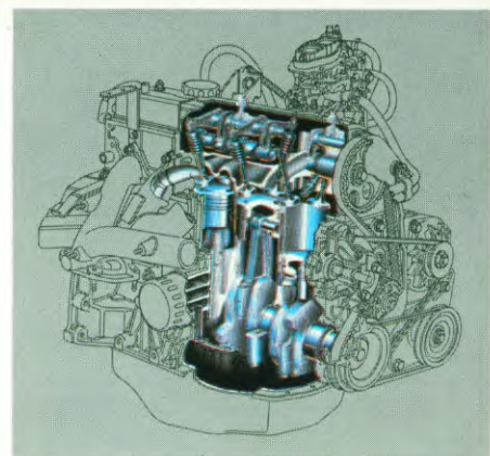
1 995 cm 3 4-cilinder benzine motor met tweetraps carburateur. Max. vermogen: 103 DIN pk bij 5500 t/min. 2 068 cm 3 4 cilinder dieselmotor. Max. vermogen: 64 DIN pk bij 4500 t/min.
