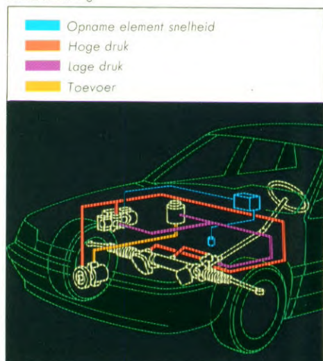
Snelheidsafhankelijke stuurbekrachtiging.
