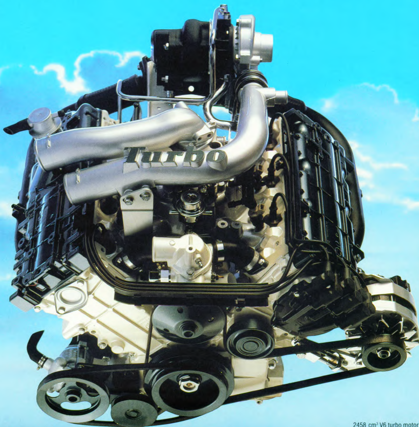
2458 cm 3 V6 turbo motor
