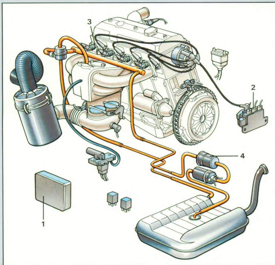
Renix elektronische brandstofinspuiting (GTX):
