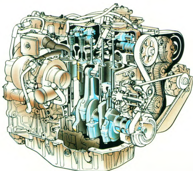
2068 cm³ turbo Diesel motor
